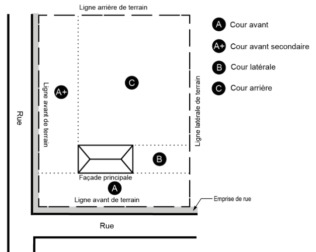
D) Terrain d'angle régulier
